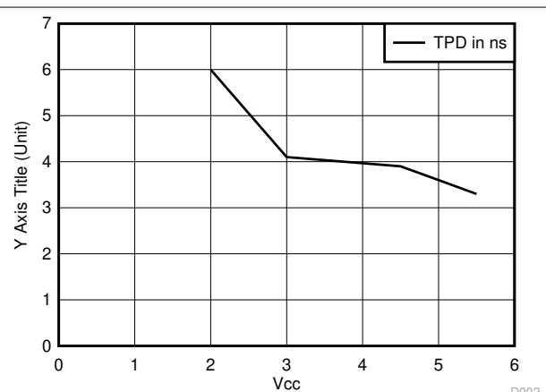
図 5-2. TPD vs V_{CC} at 25^\circ\text{C}
