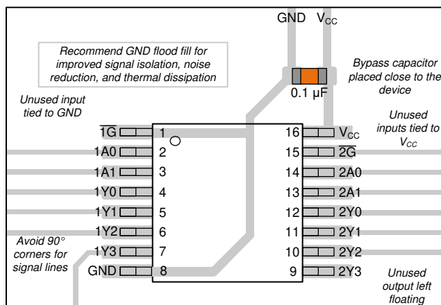
図 8-3. SN74AHC139-Q1 のレイアウト例
