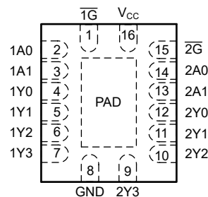
図 4-2. WBQB パッケージ、 16 ピン TSSOP (上面図)
