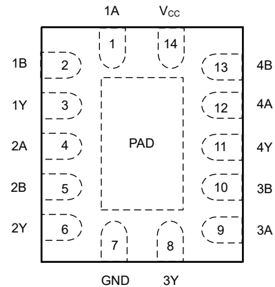
図 3-2. SN74ACT86 BQA パッケージ (透明上面図)
