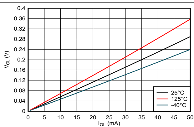
図 5-2. Low 状態における出力電圧と電流の関係、5V 電源
