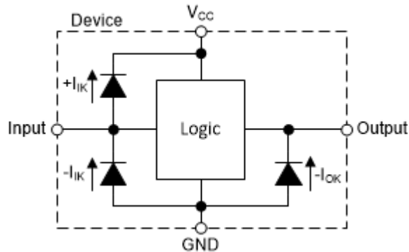
図 7-3. 各入力とオープンドレイン出力に対するクランプダイオードの電氣的配置
