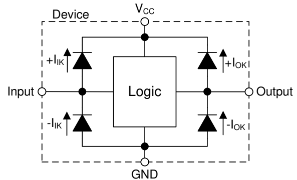
図 7-4. 各入力とプッシュプル出力に対するクランプダイオードの電氣的配置
