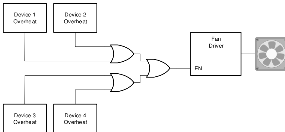
図 8-1. 代表的なアプリケーション回路図
