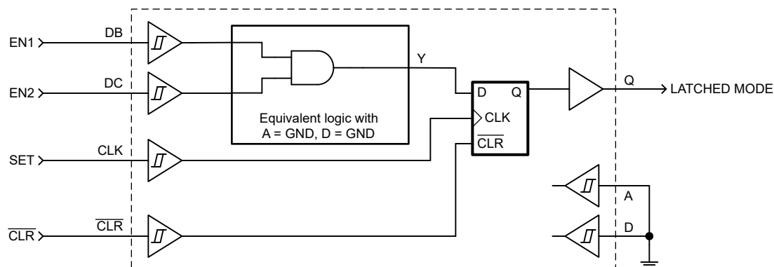
図 8-1. 代表的なアプリケーション回路図
