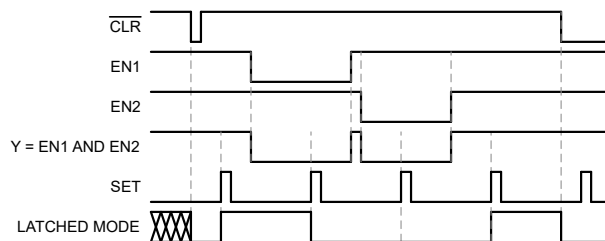
図 8-2. 代表的なアプリケーションのタイミング図
