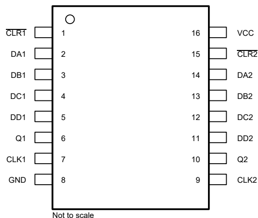
図 4-2. PW パッケージ、16 ピン TSSOP (プレビュー) (上面図)
