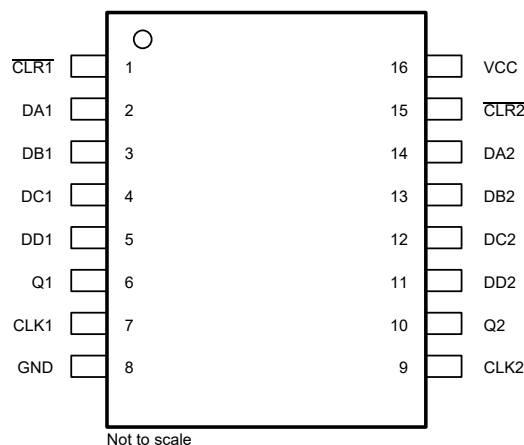
図 4-2. PW パッケージ、16 ピン TSSOP (レビュー) (上面図)
