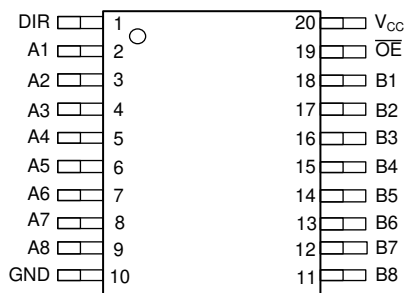
図 4-1. DGS および PW パッケージ、 20 ピン VSSOP および TSSOP (上面図)
