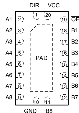
図 4-2. RKS パッケージ、 20 ピン VQFN (上面図)
