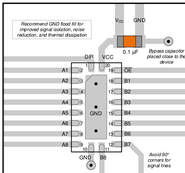
図 8-3. SN74ACT245-Q1 のレイアウト例
