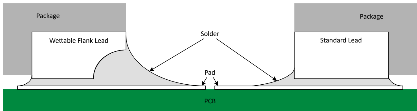
図 7-1. 半田付け後のウェットابل フランク QFN パッケージと標準 QFN パッケージの概略断面図
