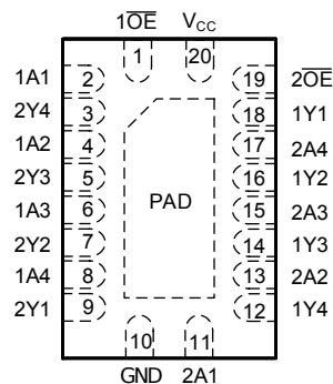
図 4-2. SN74ACT240-Q1 VQFN パッケージ (上面図)
