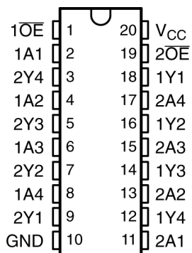
図 4-1. SN74ACT240-Q1 DGS または PW パッケージ、20 ピン VSSOP または TSSOP (上面図)
