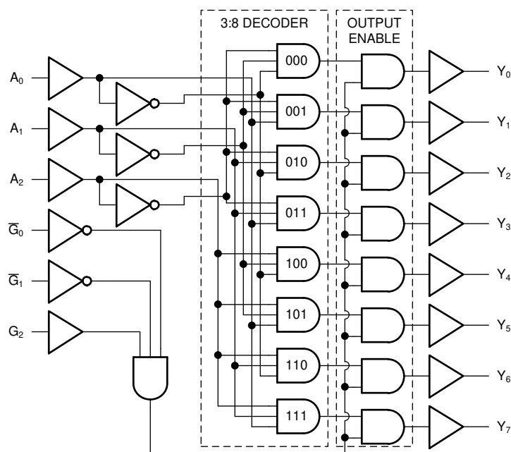
図 7-1. SN74ACT238-Q1 の論理図 (正論理)
