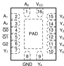
BQB パッケージ、16 ピン WQFN (透過上面図)
