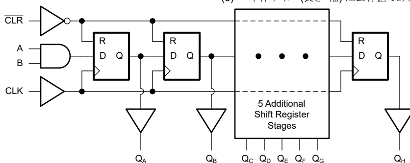
機能図
