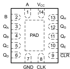
図 4-2. WBQA パッケージ 14 ピン WQFN (上面図)
