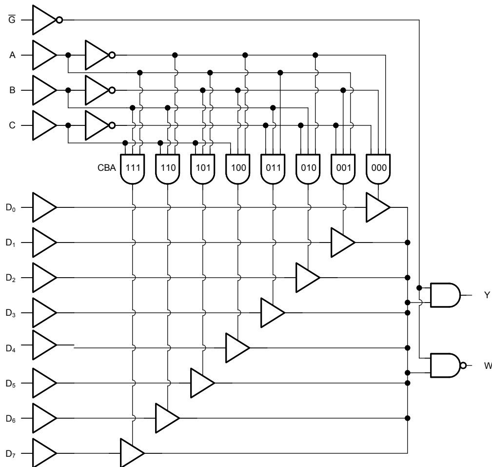
図 7-1. SN74ACT151-Q1 の論理図 (正論理)
