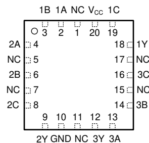
図 4-2. FK パッケージ (上面図)
