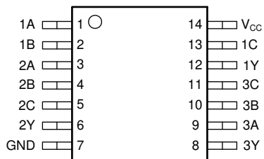
図 4-1. J または W パッケージ (上面図)
