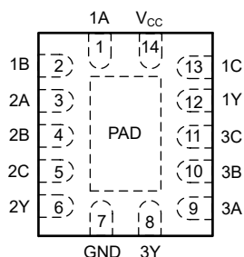
図 4-3. SN74ACT10 BQA または パッケージ (上面図)
