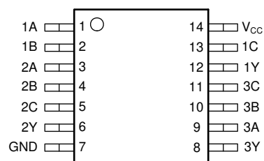
図 4-4. SN74ACT10 D、PW、N、DB パッケージ (上面図)
