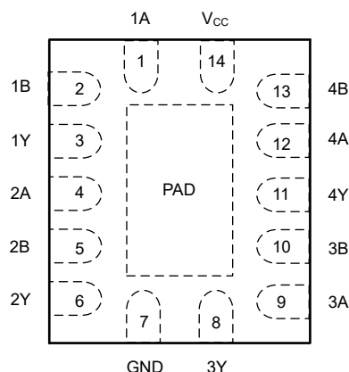
図 3-2. SN74ACT00 BQA パッケージ (透明上面図)
