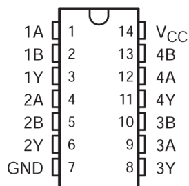
図 3-1. SN54AC86 J または W パッケージ、 SN74AC86 D、DB、N、NS、PW パッケージ (上面図)
