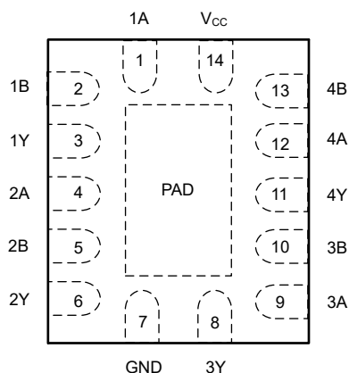
図 3-3. BQA パッケージ (上面図)
