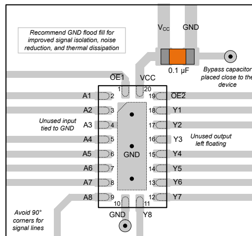
図 8-3. RKS パッケージに封止した SN74AC8541-Q1 のレイアウト例
