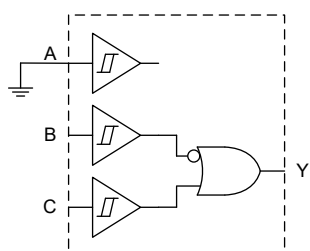
1 個の反転入力採用 2 入力 OR
