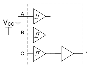
シュミット トリガ バッファ
