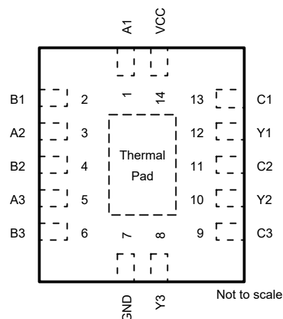
図 4-2. SN74AC3G98-Q1 BQA パッケージ、14 ピン WQFN (上面図)
