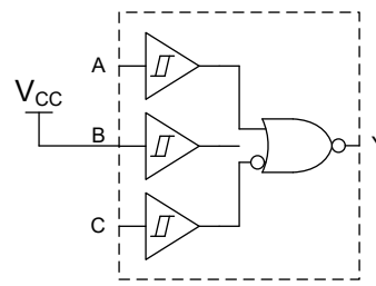
1 個の反転入力採用 2 入力 NOR
