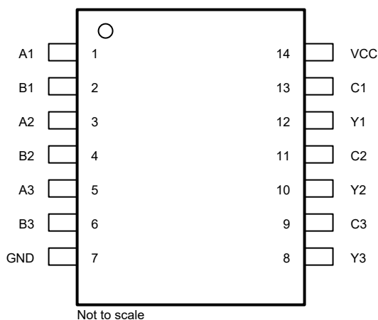
図 4-1. SN74AC3G98-Q1 PW パッケージ、14 ピン TSSOP (上面図)
