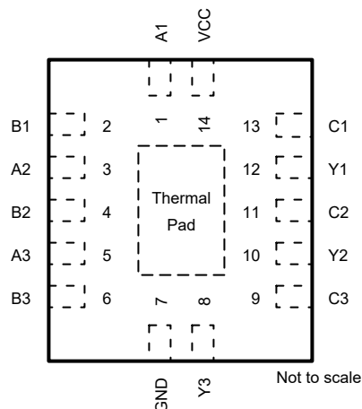
図 4-2. SN74AC3G97 BQA パッケージ、14 ピン WQFN (上面図)
