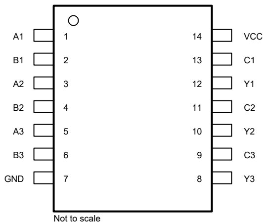
図 4-1. SN74AC3G97 PW パッケージ、14 ピン TSSOP (上面図)
