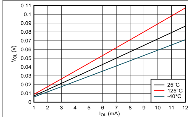
図 5-9. Low 状態における出力電圧と電流との関係、3.3V 電源
