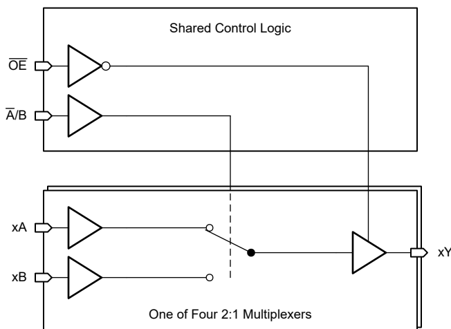
ロジック図
