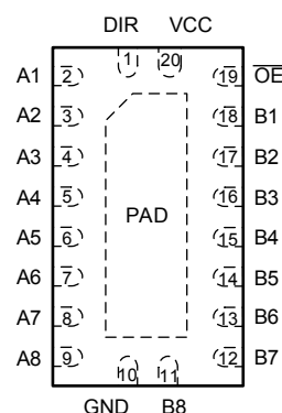
図 4-2. RKS パッケージ、20 ピン VQFN (上面図)
