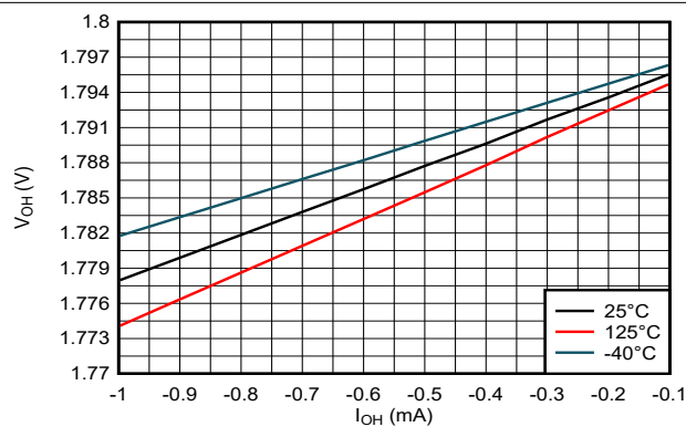
図 5-12. HIGH 状態での出力電圧と電流との関係、1.8V 電源
