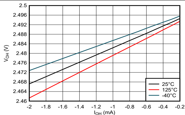
図 5-10. HIGH 状態での出力電圧と電流との関係、2.5V 電源
