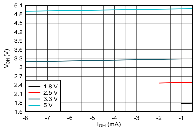
図 5-4. HIGH 状態での出力電圧と電流との関係
