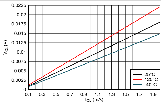
図 5-11. LOW 状態での出力電圧と電流との関係、2.5V 電源
