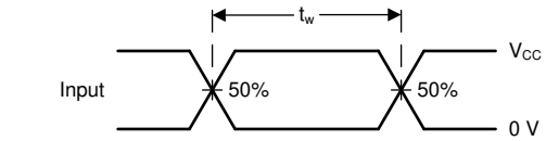
図 6-2. 電圧波形、パルス幅
