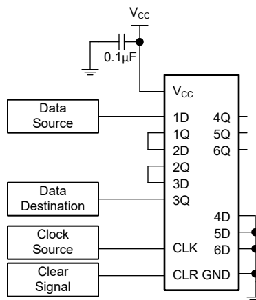
図 8-1. 代表的なアプリケーションのブロック図
