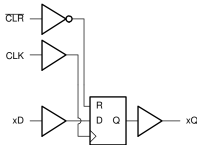
図 7-1. SN74ACT164-Q1 の論理図 (正論理)
