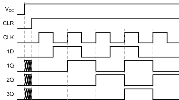
図 8-2. アプリケーション タイミング図
