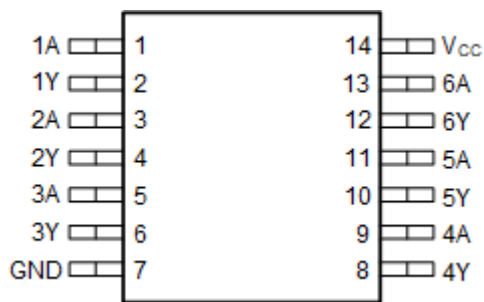
図 4-1. SN74AC16-Q1 PW パッケージ、14 ピン TSSOP (上面図)
