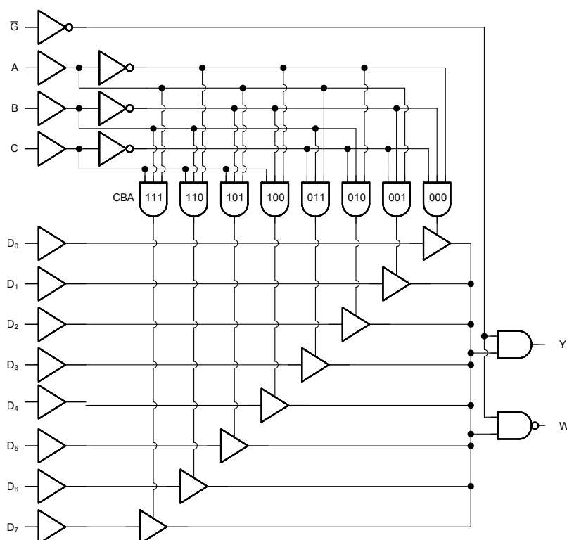
ロジック図
