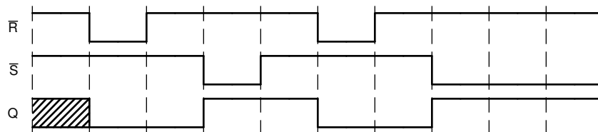
図 8-2. アプリケーションのタイミング図
