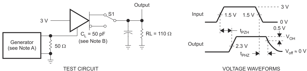
図 6-3. ドライバテスト回路と電圧波形
