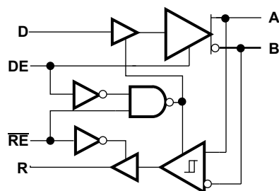
論理図 (正論理)
