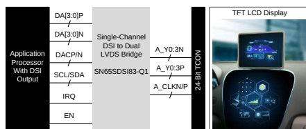
SN65DSI83-Q1回路図
