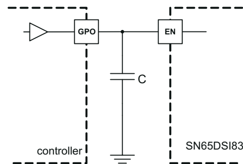
図 7-3. EN Input from Active Controller
