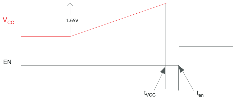
図 7-1. Cold Start V_{CC} Ramp up to EN
