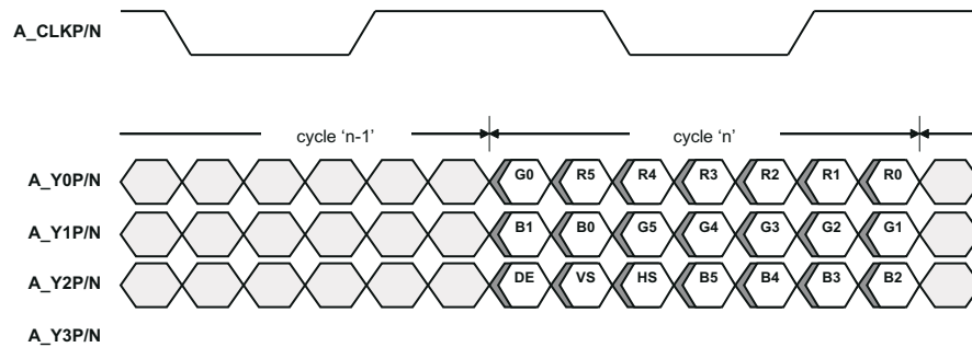
図 7-4. FlatLink Output Data; Single-Link 18 bpp
