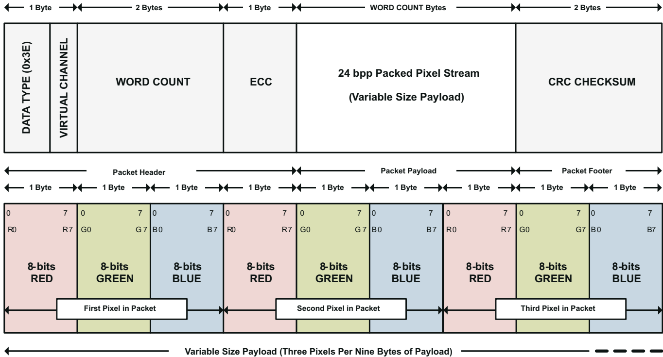
図 7-11. 24 bpp DSI Packet Structure
