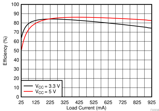
SN6505B + Würth 750315371
