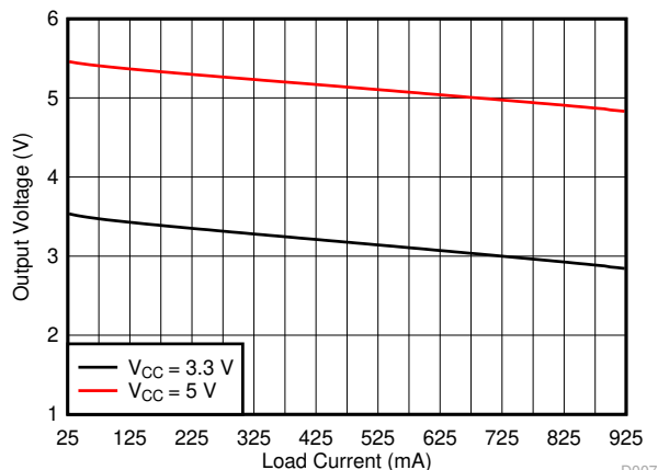
SN6505B + Würth 750315371
