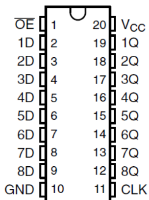
図 4-1. PW パッケージ (上面図)
