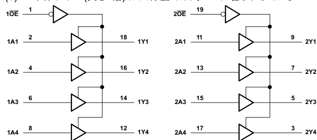
論理図 (正論理)
