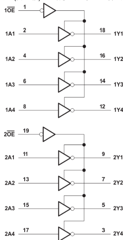
論理図 (正論理)
