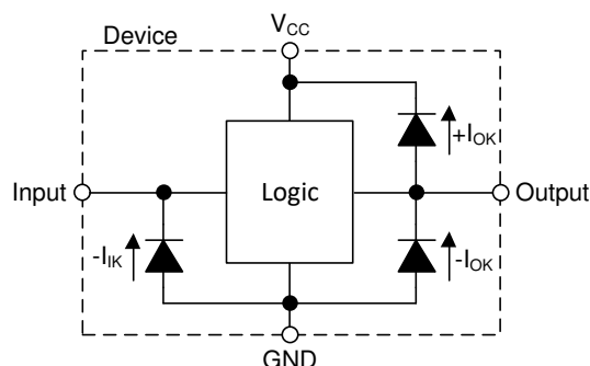
図 7-1. 各入力と出力に対するクランプ ダイオードの電气的配置
