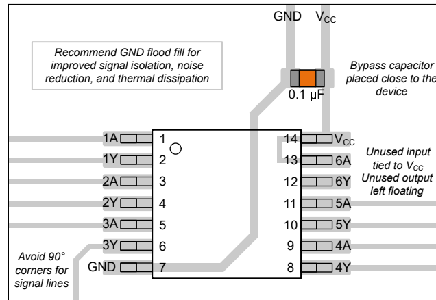
図 8-3. レイアウト例 : SN54SC6T06-SEP
