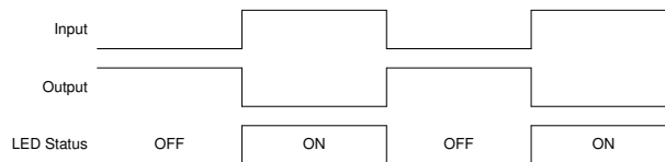
図 8-2. アプリケーション タイミング図
