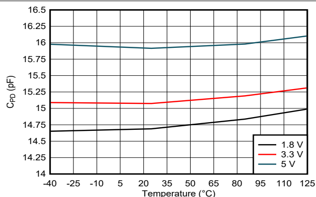
図 6-4. 温度範囲全体でのゲートごとの電力散逸容量、1.8V、3.3V、5V 電源
