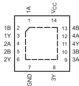
図 4-2. BQA or RGY Package 14-Pin WQFN or VQFN (Top View)
