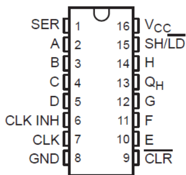
J、D、DB、N、NS、PW パッケージ 16 ピン CDIP、SOIC、SSOP、PDIP、SO、TSSOP 上面図
