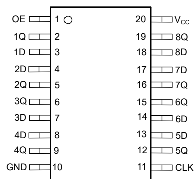
図 4-4. SN74AHCT374 PW、DW、N、DB、DGS パッケージ (上面図)
