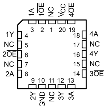
図 4-3. SN54AHCT125 FK パッケージ、(上面図)
