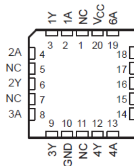
図 4-2. SN54ACT04 FK Package Top View
