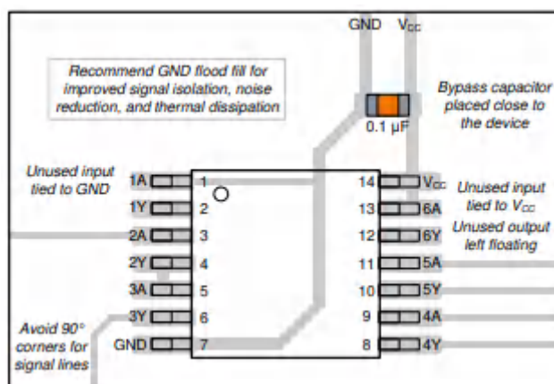
図 8-1. Layout Diagram
