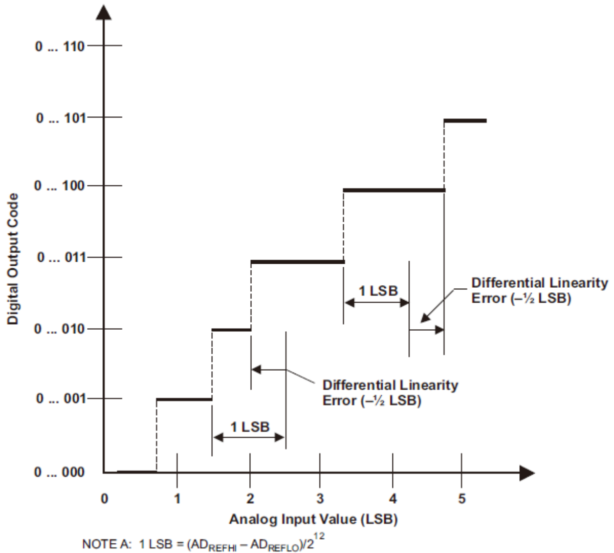
図 5-2 微分非直線性(DNL)誤差
