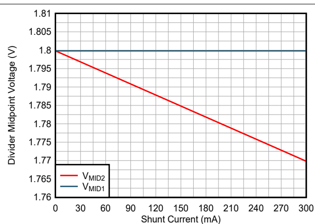
図 8-10. Simulation Result for VMID
