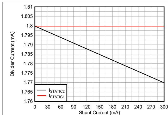
図 8-9. Simulation Result for I_{\text{STATIC}}
