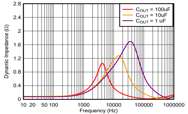
図 6-40. 出力インピーダンス
