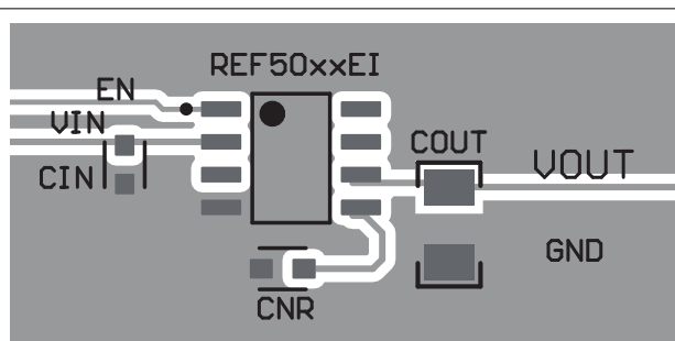
図 11-2. REF50xxEI のレイアウト例
