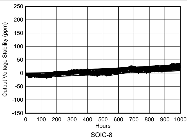
図 6-28. REF50xx の長期安定性 (最初の 1000 時間)
