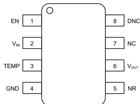
図 5-2. REF50xxEID パッケージ 8 ピン SOIC 上面図
