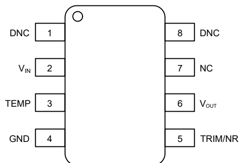
図 5-1. REF50xxAI、REF50xxID、DGK パッケージ 8 ピン SOIC、VSSOP 上面図
