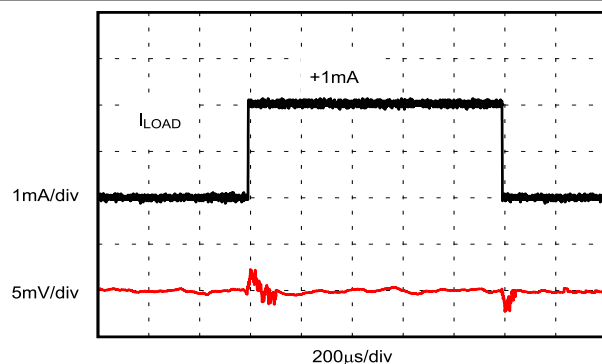
図 6-19. 負荷過渡
