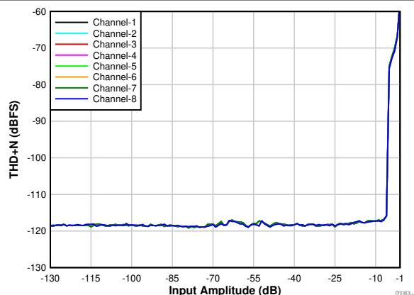
図 5-9. THD+N vs Input Amplitude
