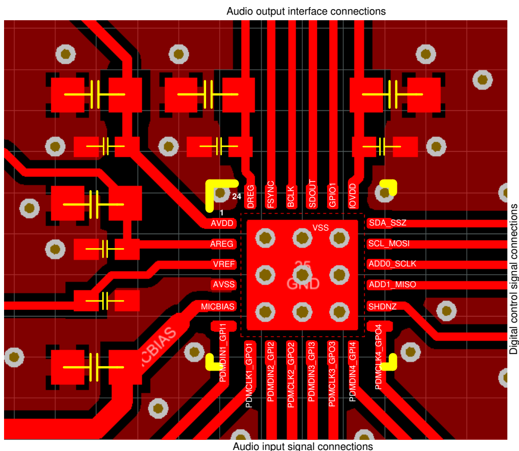
✎ 10-1. Layout Example
