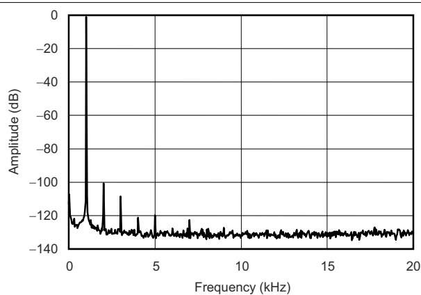
FIG 6-9. Output Spectrum
