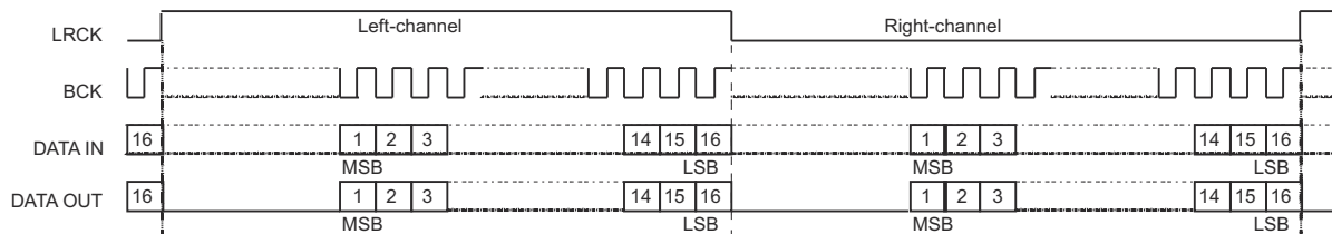
✎ 7-2. Audio Data Input/Output Format
