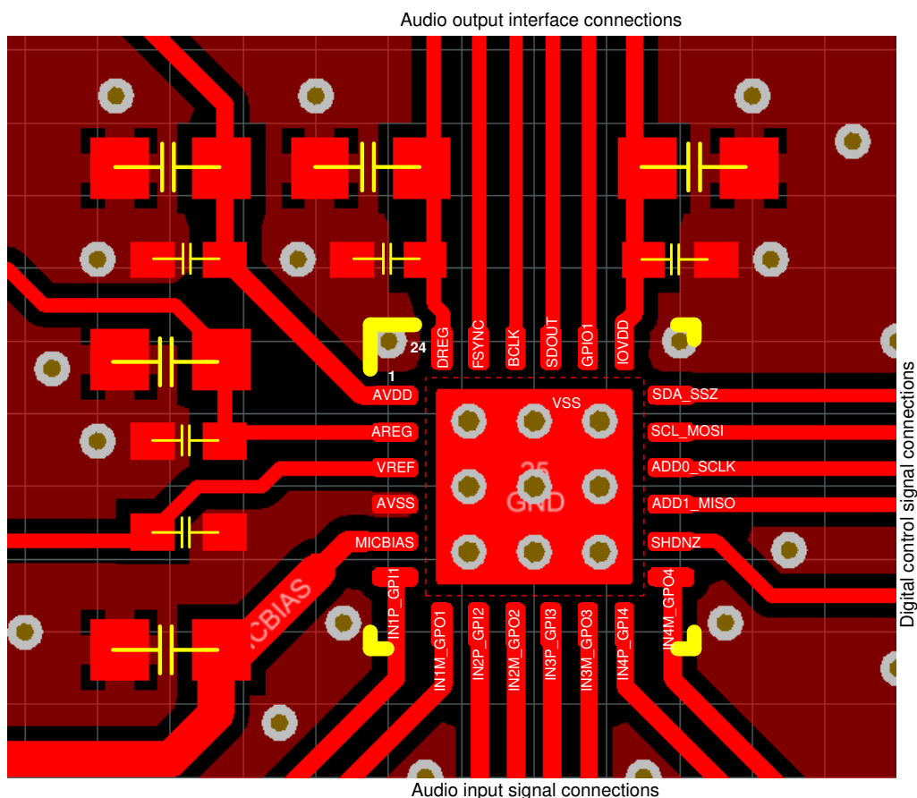
図 11-1. Layout Example
