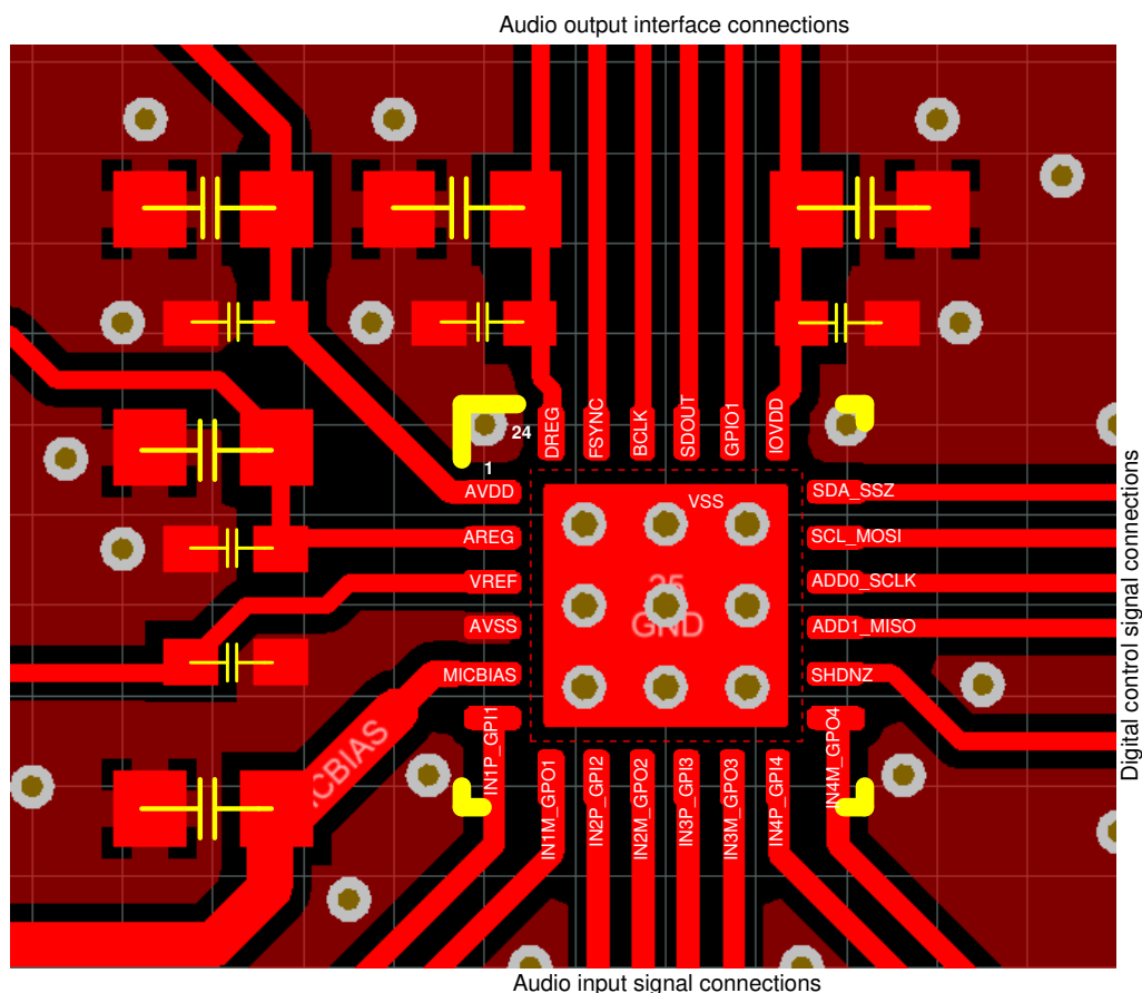
図 10-1. Layout Example
